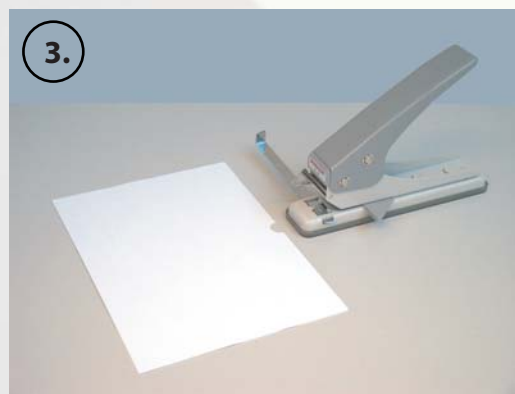
3. Papier mit gestanztem Daumenloch entnehmen
